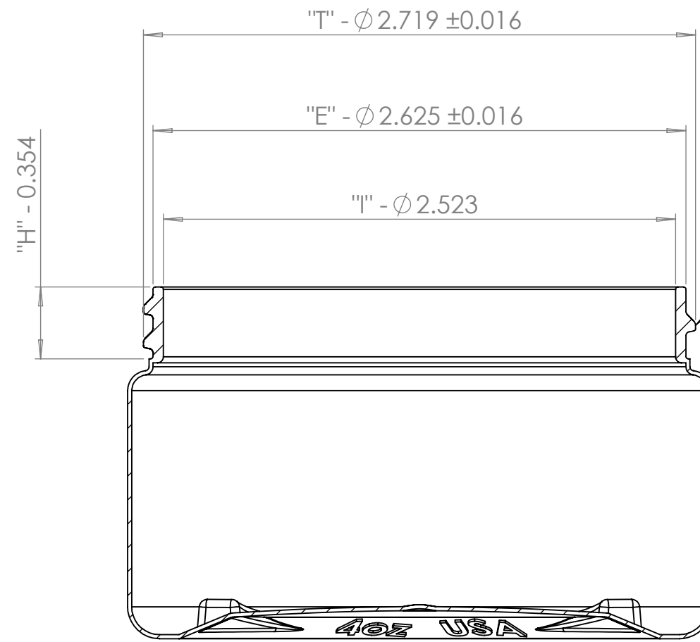
SECTION A-A
